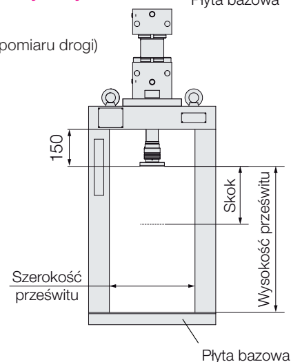
Płyta bazowa
