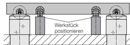
Pneumatische Auflagekontrolle
